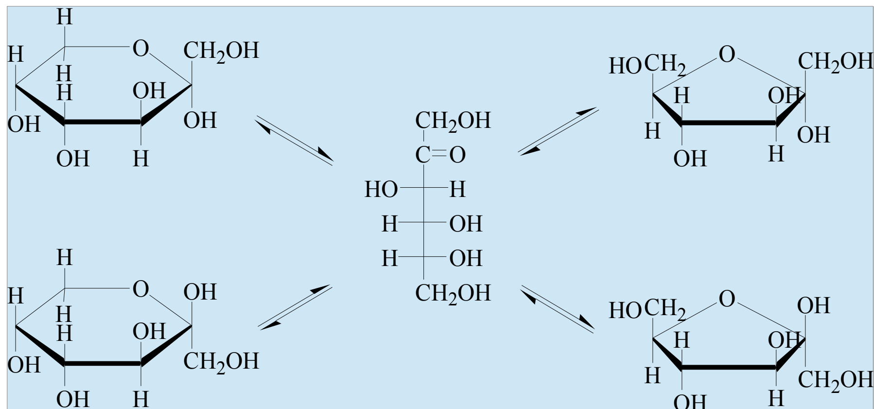
\beta -D- 吡喃果糖
