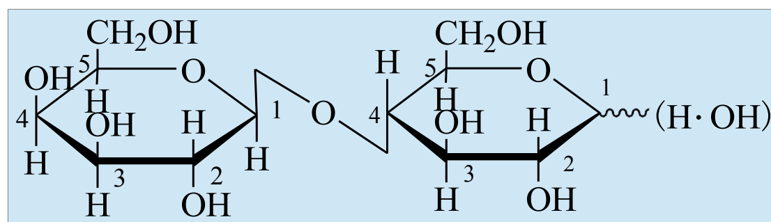
乳糖 [4-O- ( \beta -D- 吡喃半乳糖基 ) -D- 吡喃葡萄糖 ]
