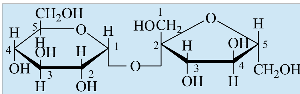
\alpha -D- 吡喃葡萄糖部分 \beta -D- 呋喃果糖部分
