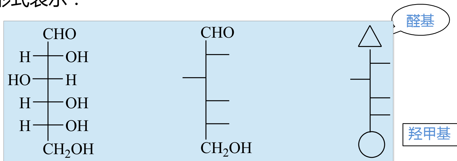
D-（+）-葡萄糖
