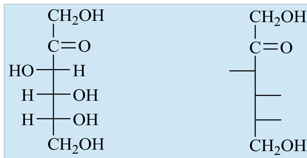
D-（-）-果糖
