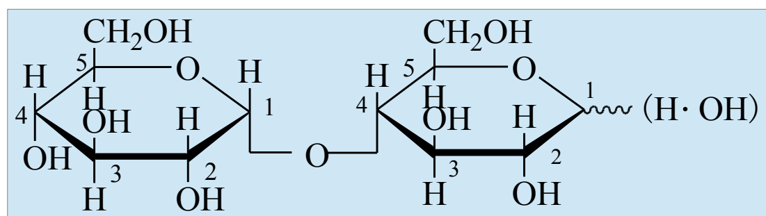
麦芽糖 [4-O- ( \alpha -D- 吡喃葡萄糖基 ) -D- 吡喃葡萄糖]
