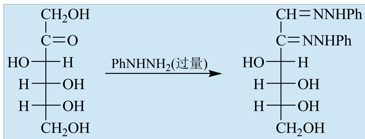
D- 果糖
